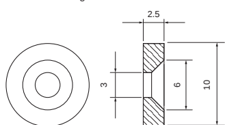
Dimensioni Magnete 300-MA
